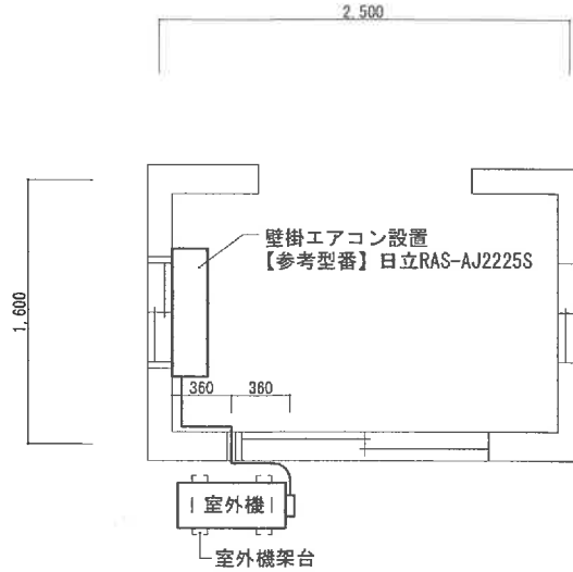
空調機設置平面図 S=1:50
