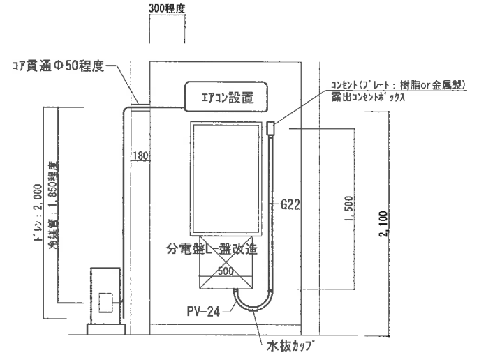
空調機設置及び電気改修立面図 S=1:50
