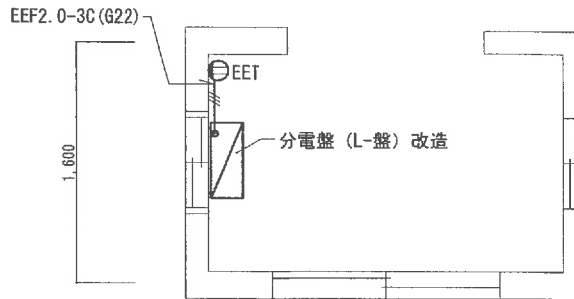
電気設備改修平面図 S=1:50
