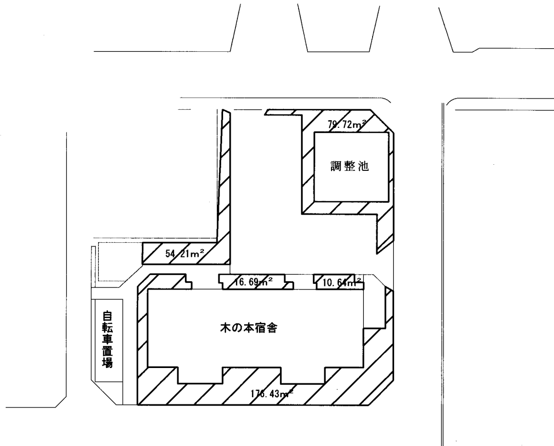
木の本宿舎配置図 S=1/500
