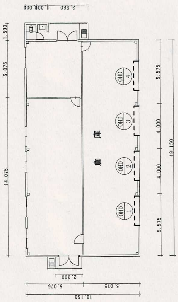
125号建物平面図 S=1:150
