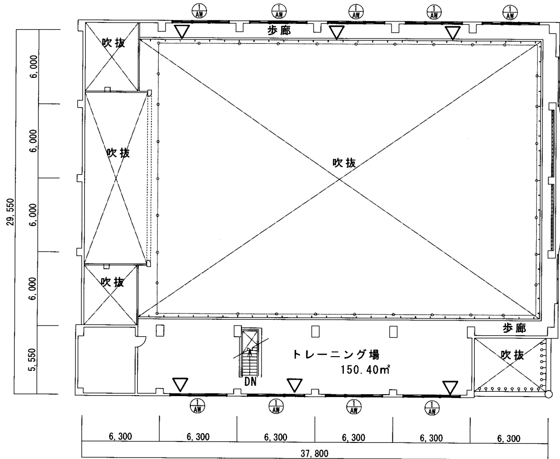
112号建物3階平面図 S=1/300
