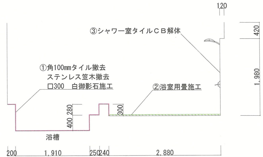
A-A' 断面図
