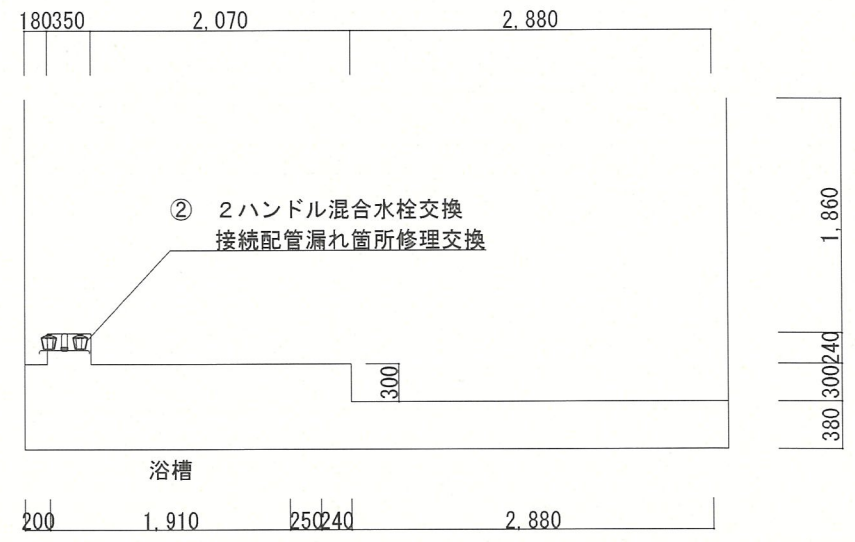
B-B' 断面図
