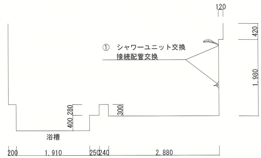
B-B' 断面図
