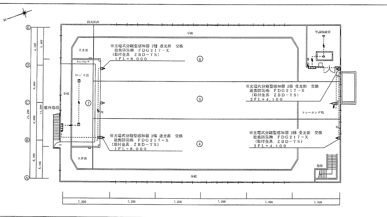
光電式分離型感知器配置図 S=1/250
