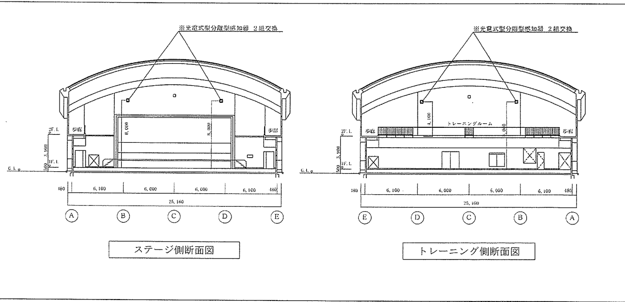
体育館断面図 S=1/300
