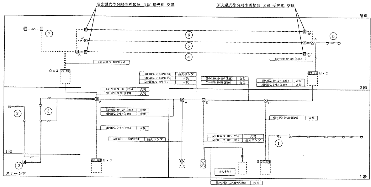
火災報知設備 系統図
