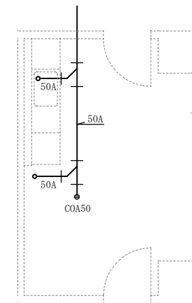
調理室平面詳細図 S=1/100
