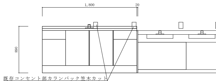
洗面台及び流し台（取替後）立面図 S=1:30
