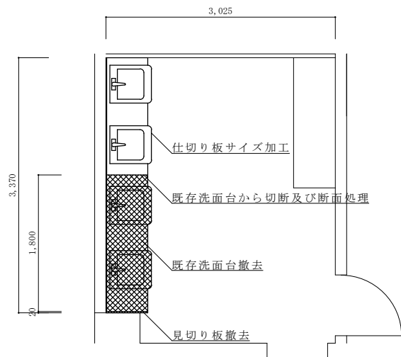
洗面台（取替前）平面図 S=1:50
