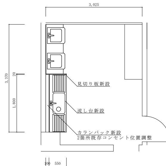
洗面台及び流し台（取替後）平面図 S=1:50
