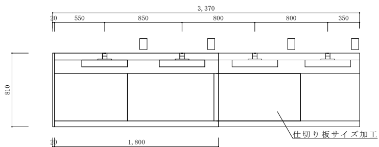
洗面台（取替前）立面図 S=1:30
