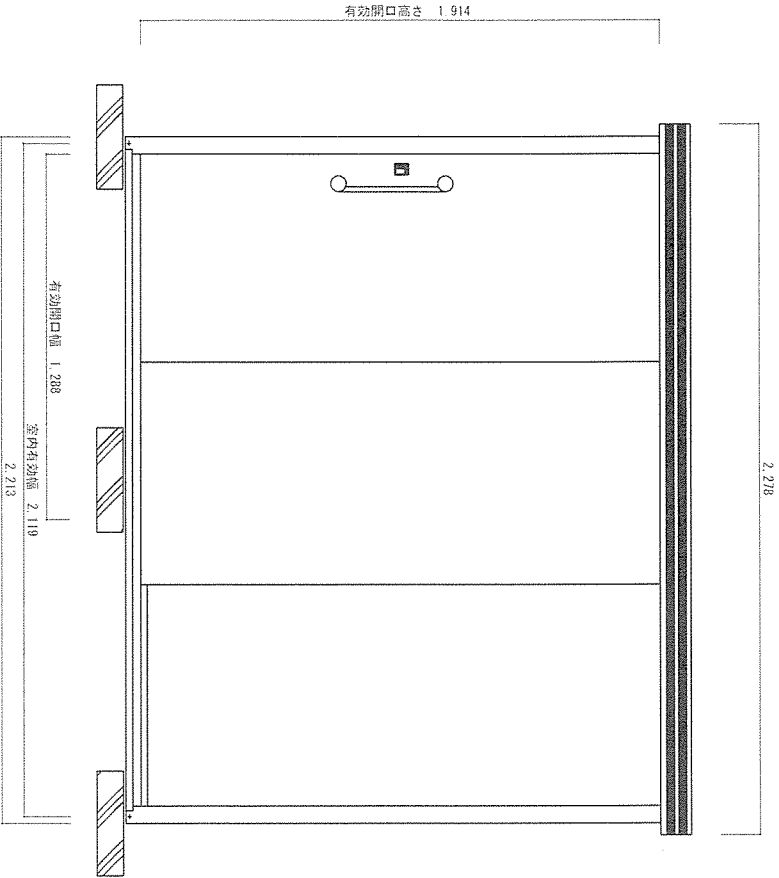
物置正面標準図
