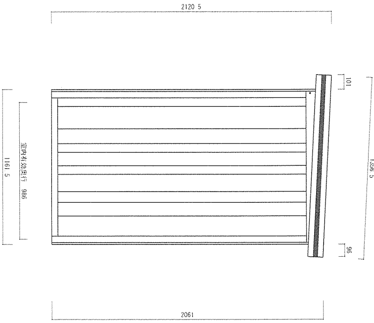
物置側面標準図
