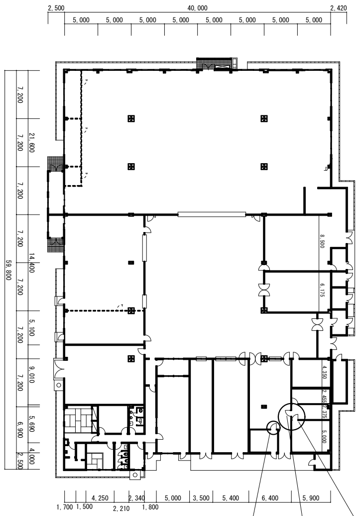
195号建物平面図 1/400
