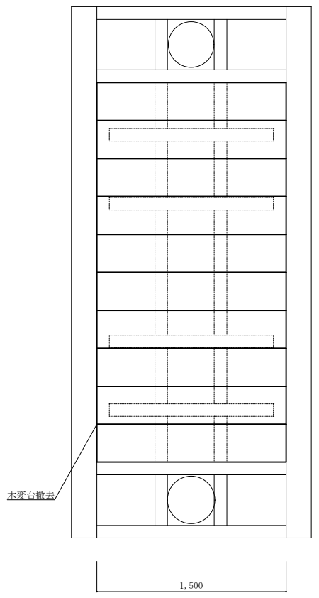
変台詳細図 (施工前) S=1:30
