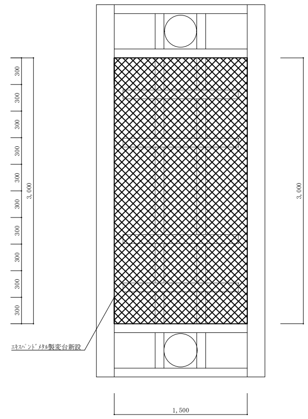
変台詳細図 (施工後) S=1:30
