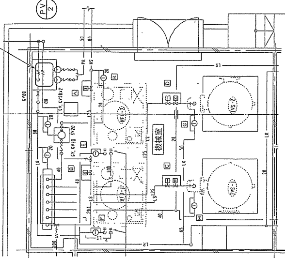
浴場機械室平面図 S=1:X
