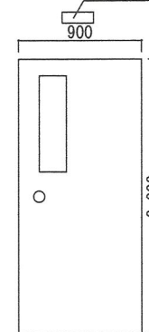
既設・新設扉図 1/50
