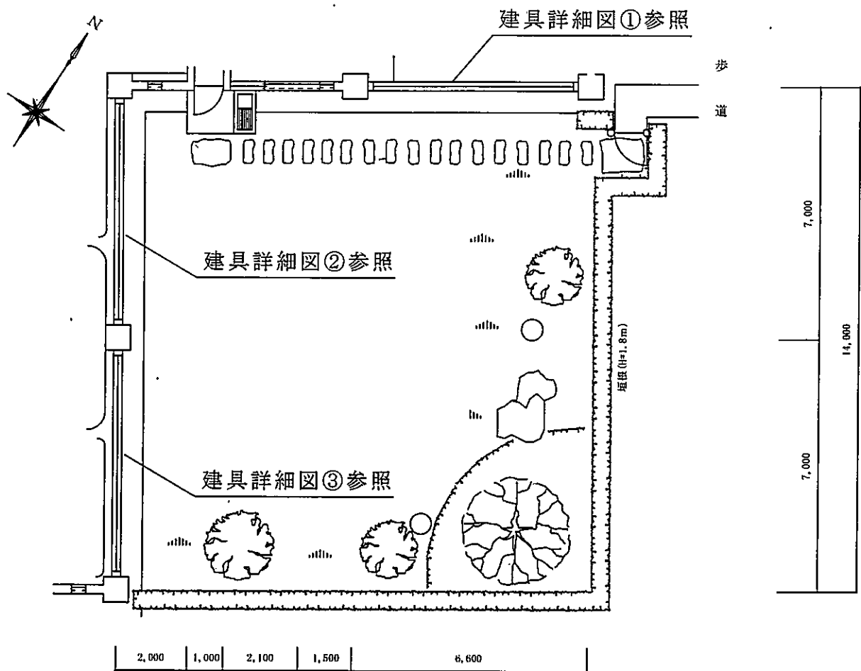
262号建物平面図 S=1/150
