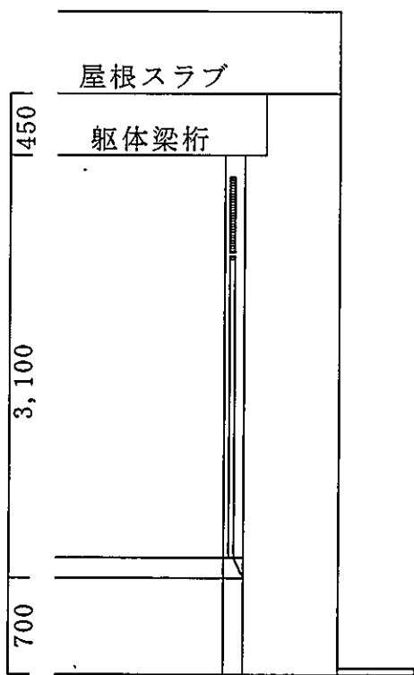
建具断面図 (取付前) S=1/50
