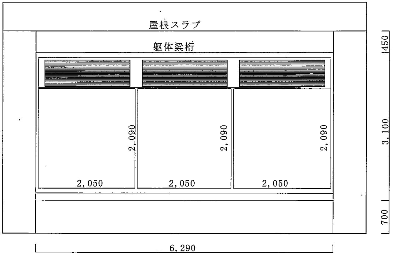
建具詳細図② S=1/50
