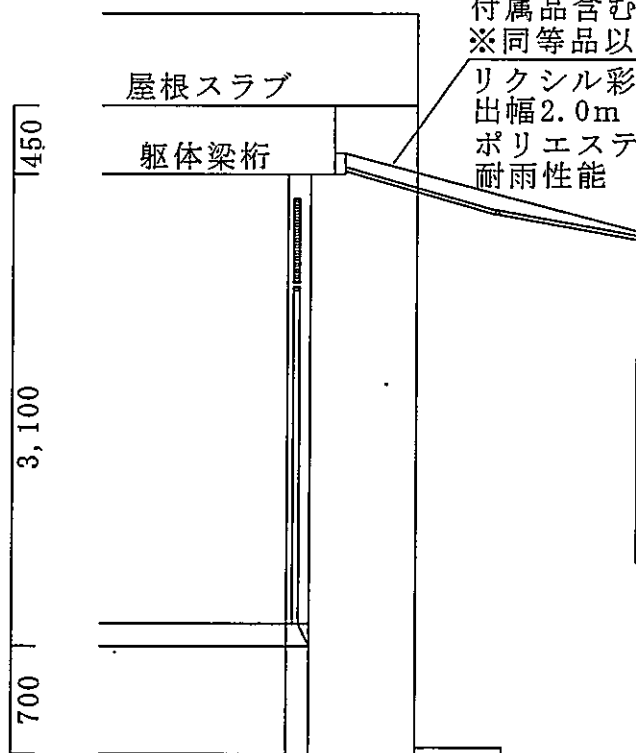
建具断面図 (改修前) S=1/50
