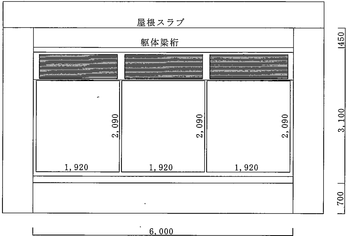
建具詳細図① S=1/50
