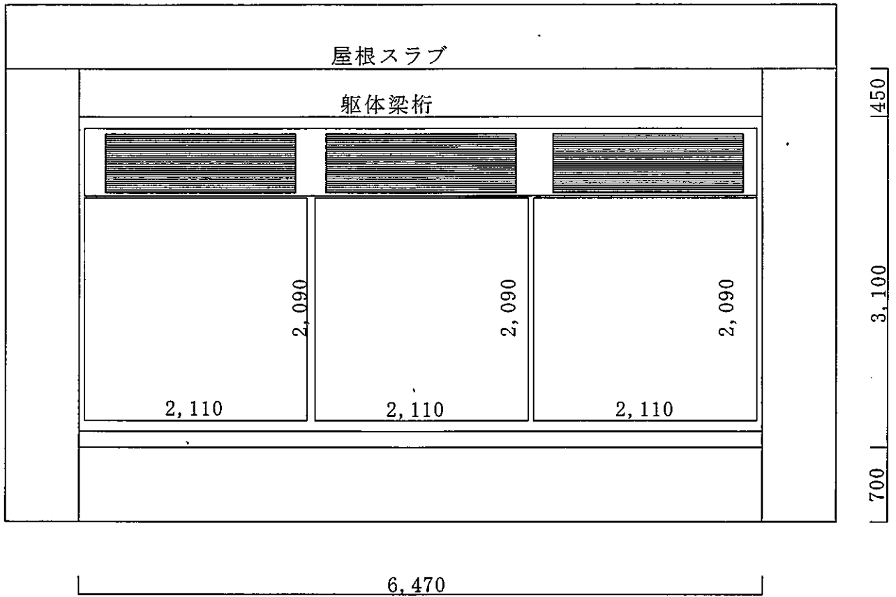
建具詳細図③ S=1/50
