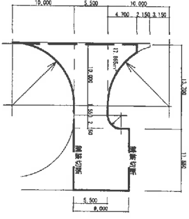
①727M舗装修理箇所詳細図 S=1:600
