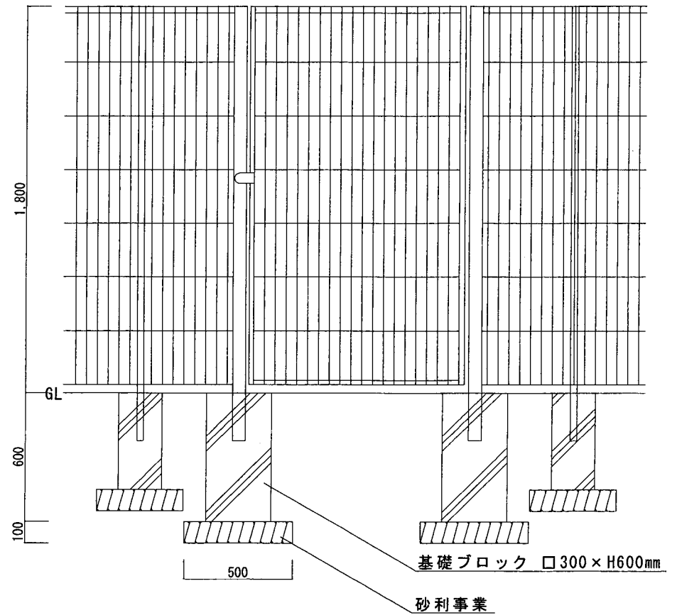
スチールメッシュ門扉部分断面図 S=1/25
