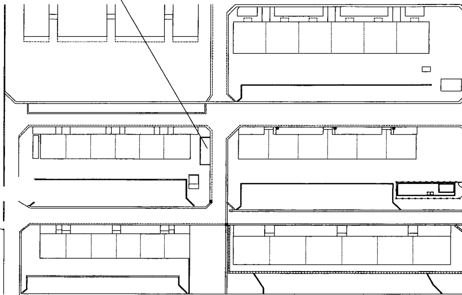
配置図 S=1/1,000
