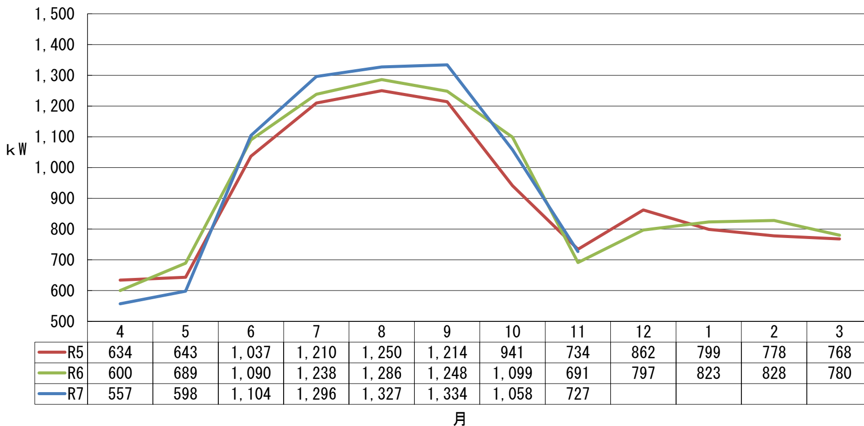
年度別 月別最大デマンド値曲線 (電力供給業者データ使用)
