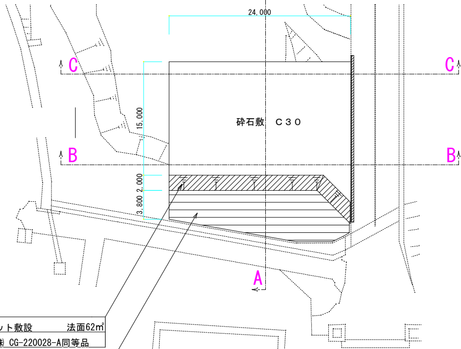
施工後配置図 S=1/500
