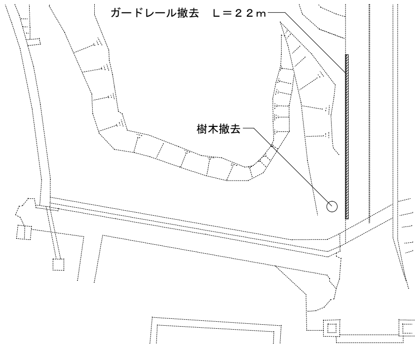
施工前配置図 S=1/500
