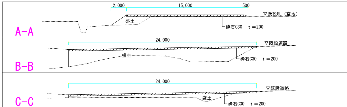
断面図 S=1/300
