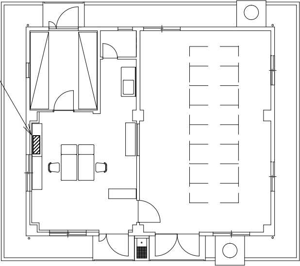
205号建物平面図 S = 1 / 200
