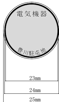
製作図
