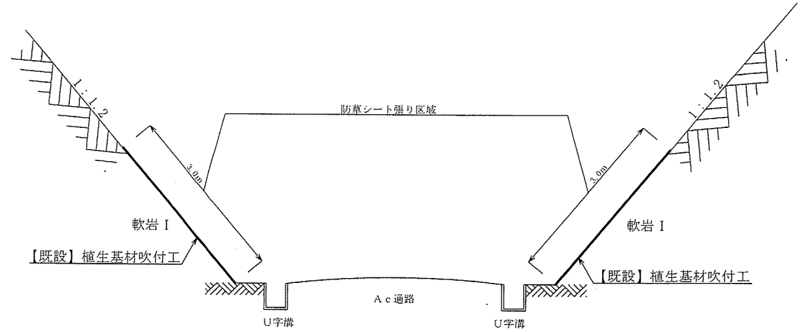
現地断面図 S=1/60
