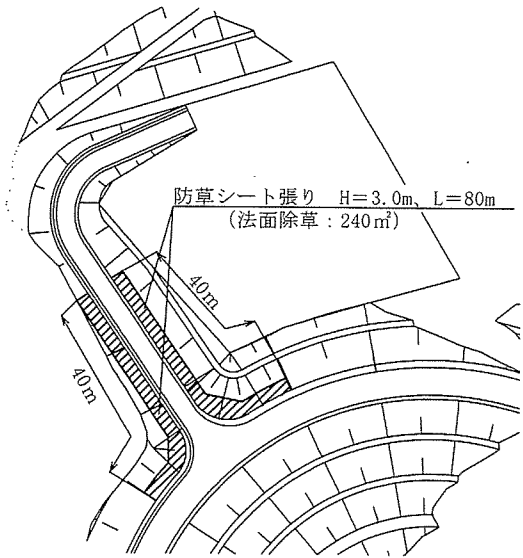
防草シート配置図 S=1/1,000
