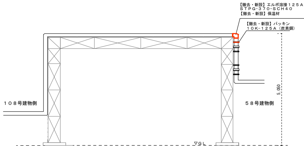
立面図
