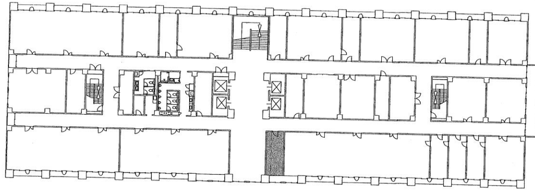
1号建物5階平面図 S=1/600
