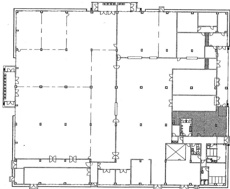
97号建物1階平面図 S=1/600
