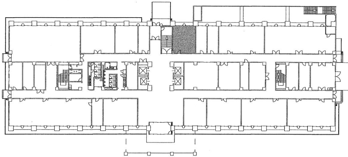
1号建物1階平面図 S=1/600
