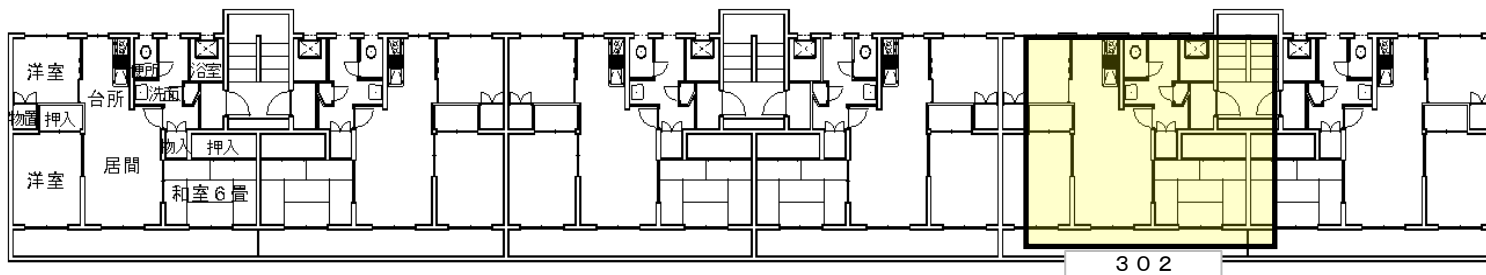
新川宿舎平面図 (基準階)
