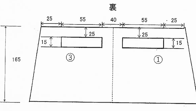
付図2-形状及び寸法等
