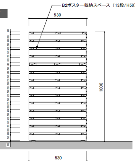
E断面
