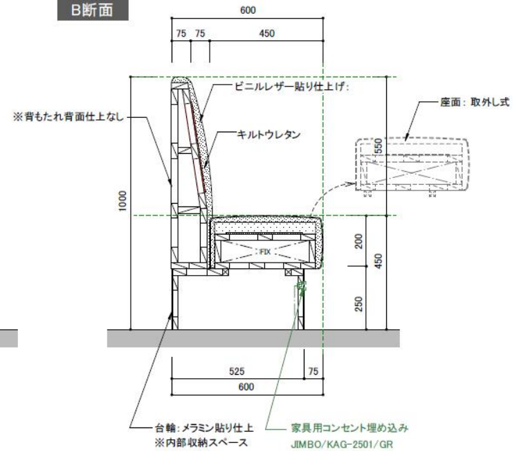
B断面
