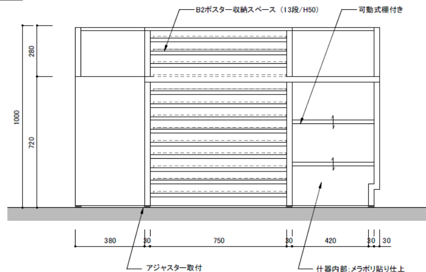
B立面
