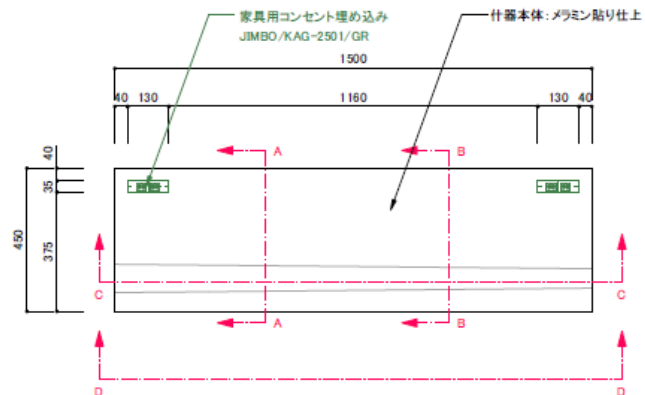
平面图
