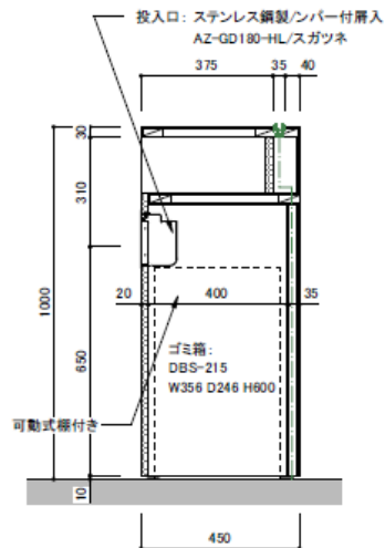
A断面
