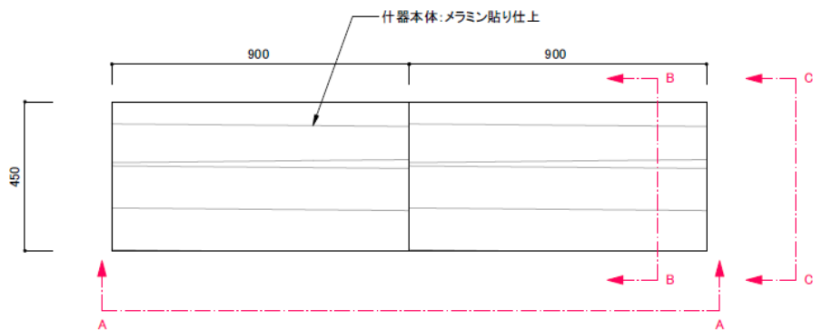
平面図
