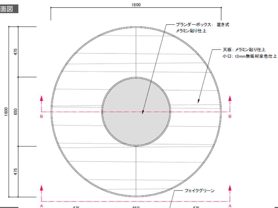
A立面
