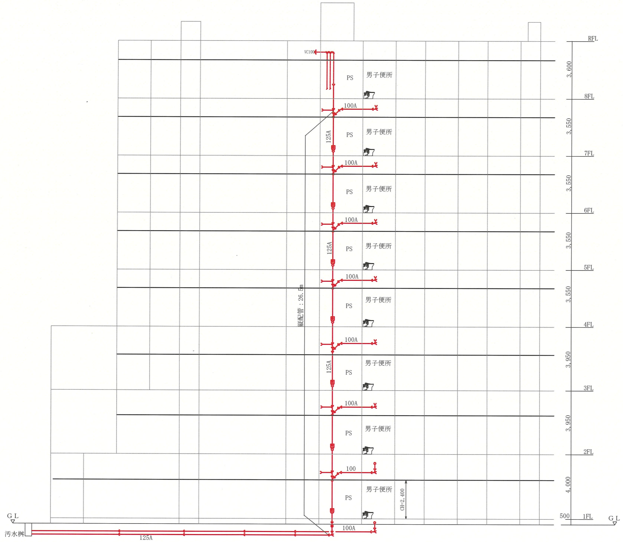
汚水配管系統図 S=1/200
