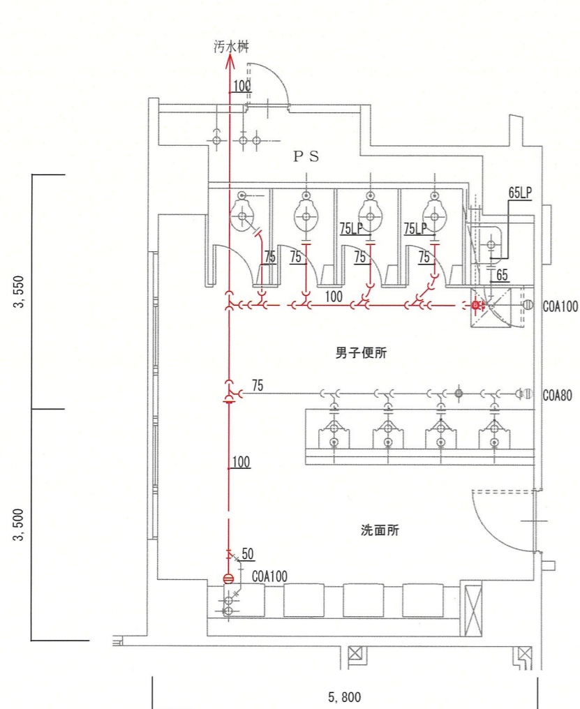
1階便所污水配管詳細図 S=1/80
