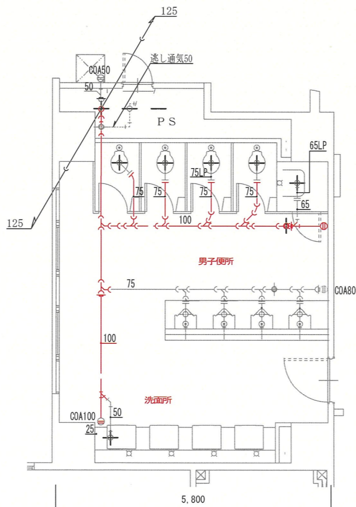
2～3階便所污水配管詳細図 S=1/80
