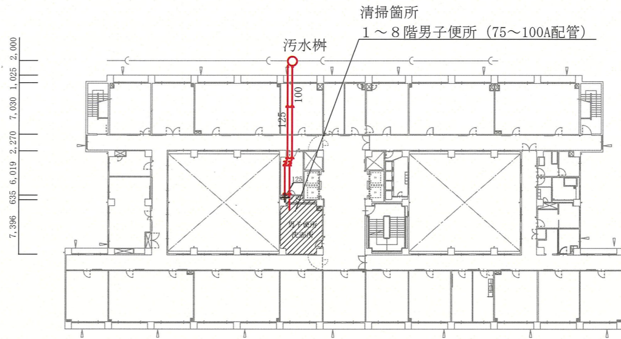
1階便所污水配管図 S=1/500
