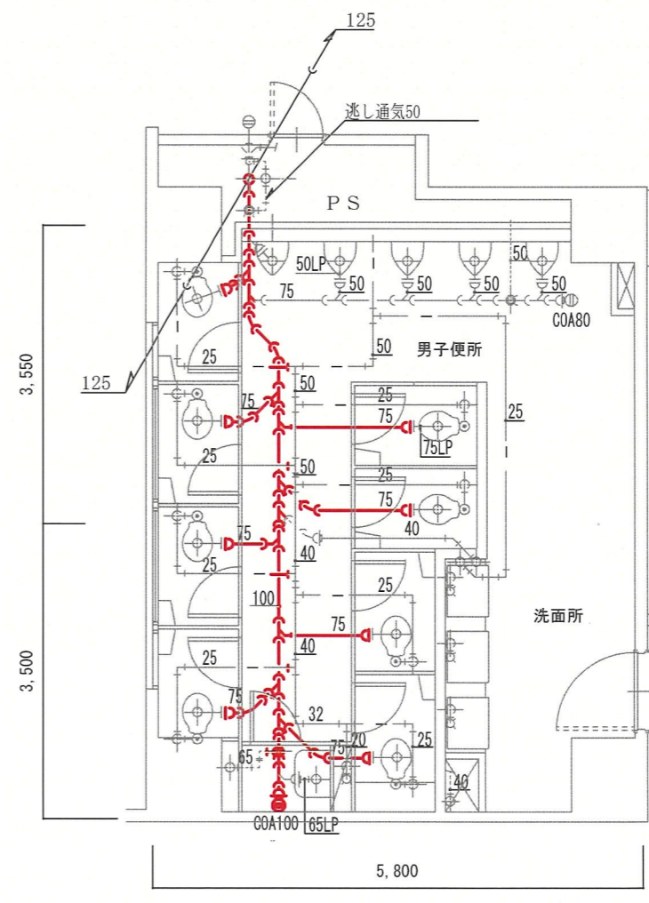
4～8階便所污水配管詳細図 S=1/80
