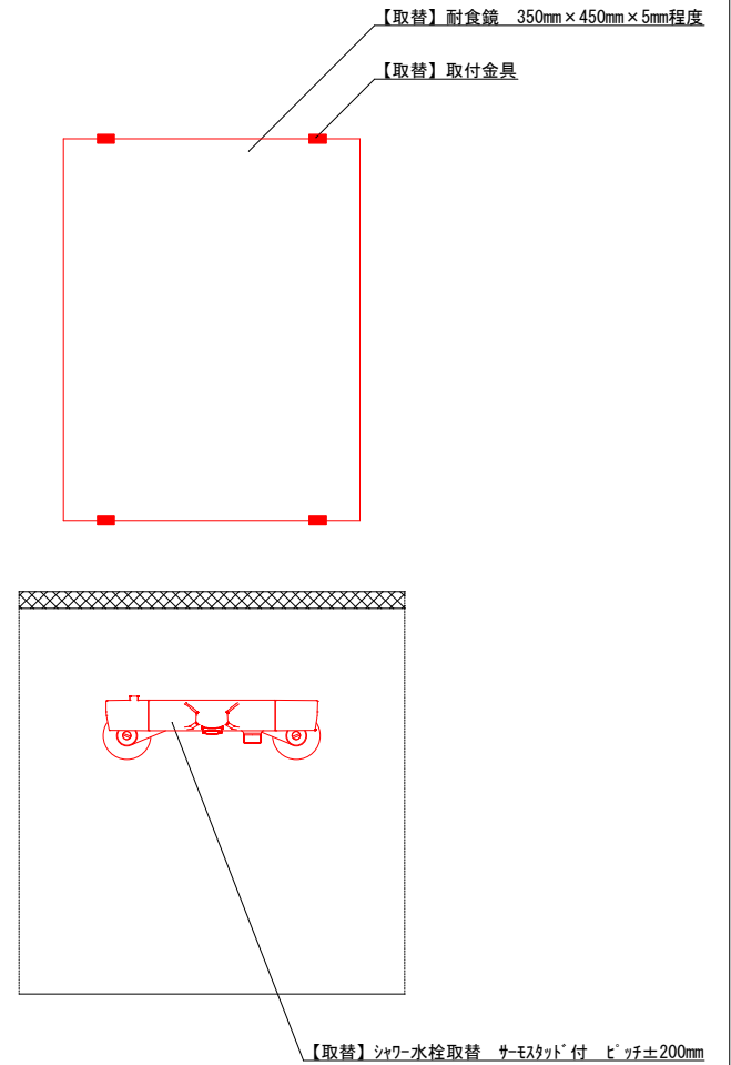
耐食鏡・シャワー水栓標準図 S=1/X
