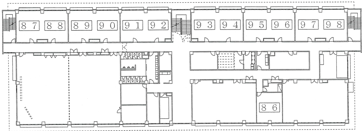
135号建物【5階】 平面図 S=1/350
