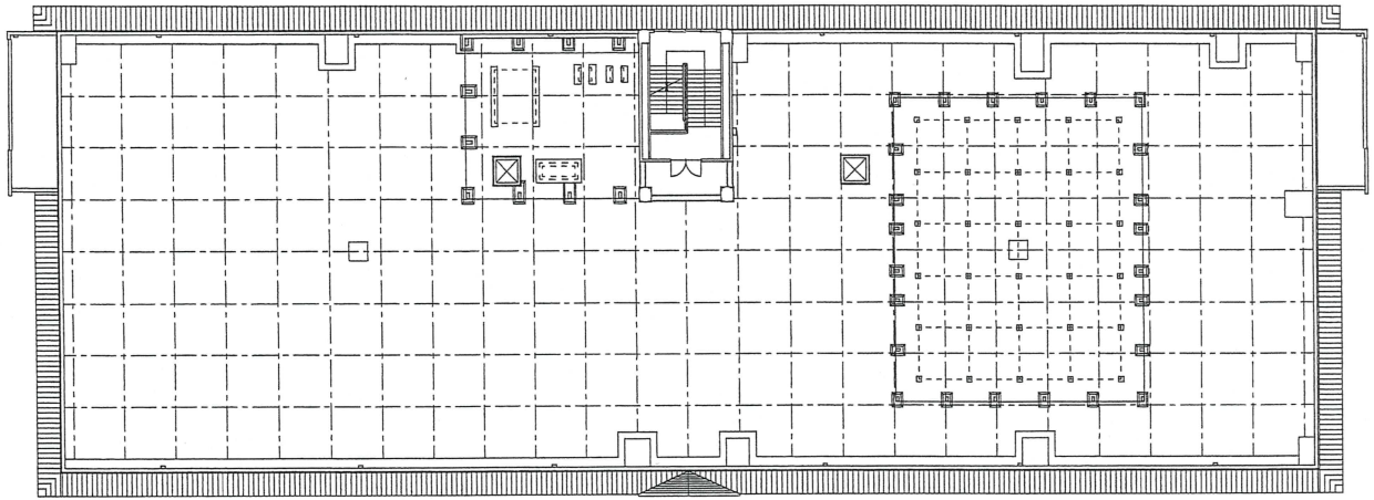
135号建物【RF階】 平面図 S=1/350
