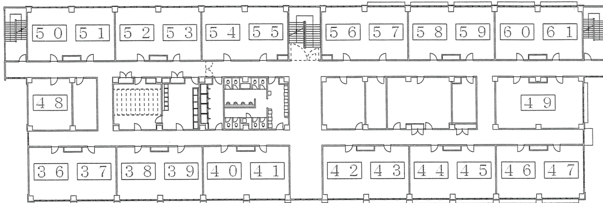
135号建物【3階】 平面図 S=1/350
