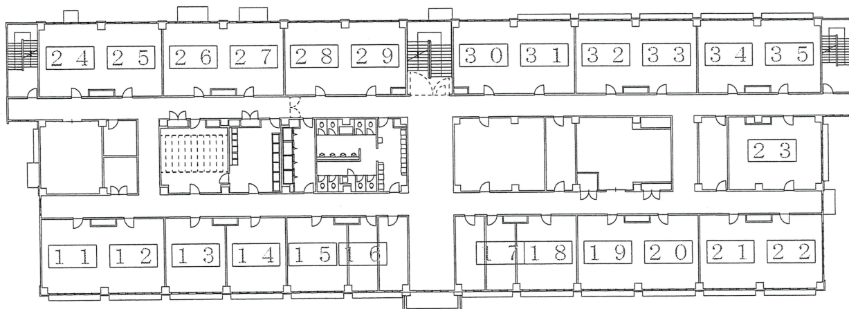
135号建物【2階】 平面図 S=1/350
