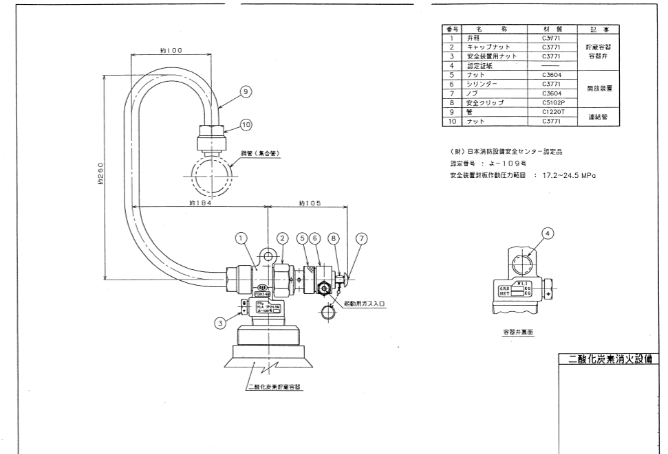
三国山貯蔵容器弁詳細図 S=1:N
