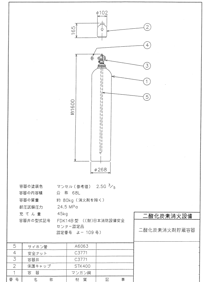
三国山貯蔵容器姿図 S=1:N
