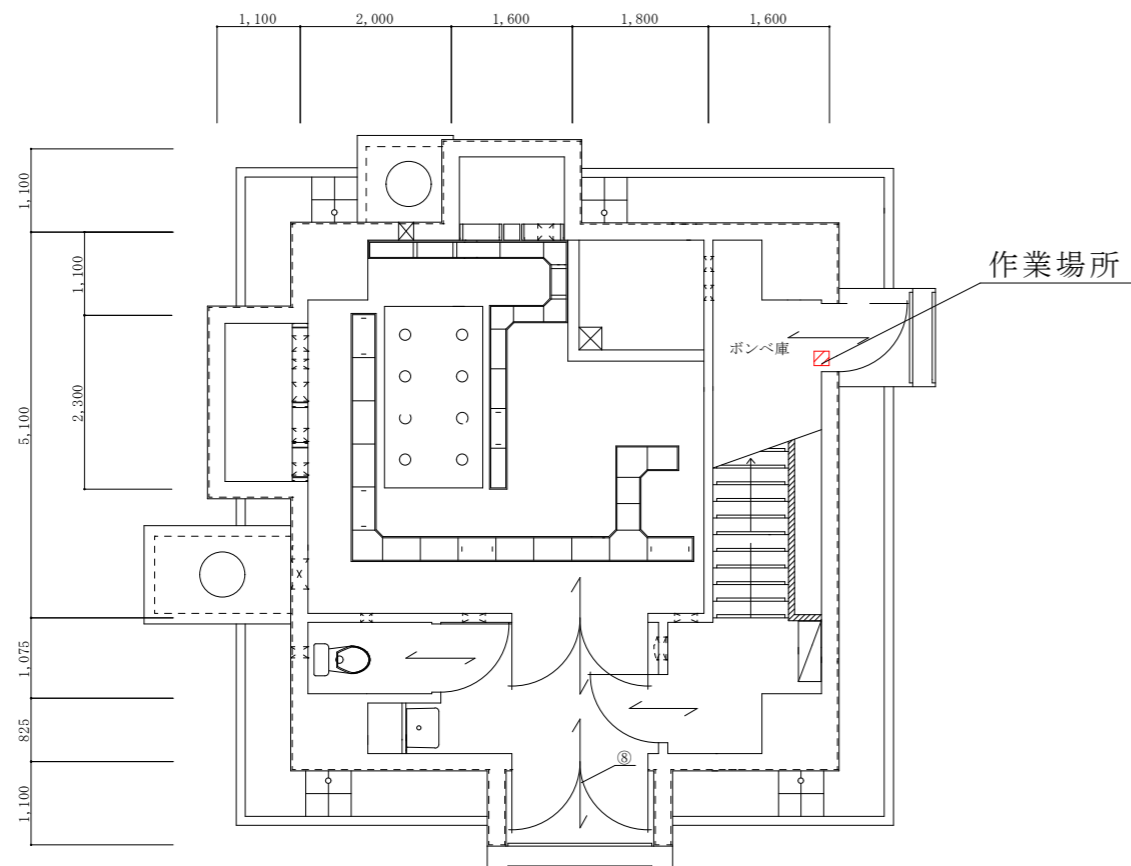
三国山1階平面図 S=1:100
