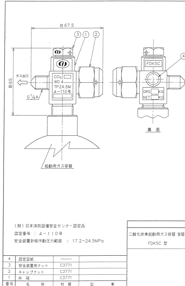
三国山起動容器弁詳細図 S=1:N
