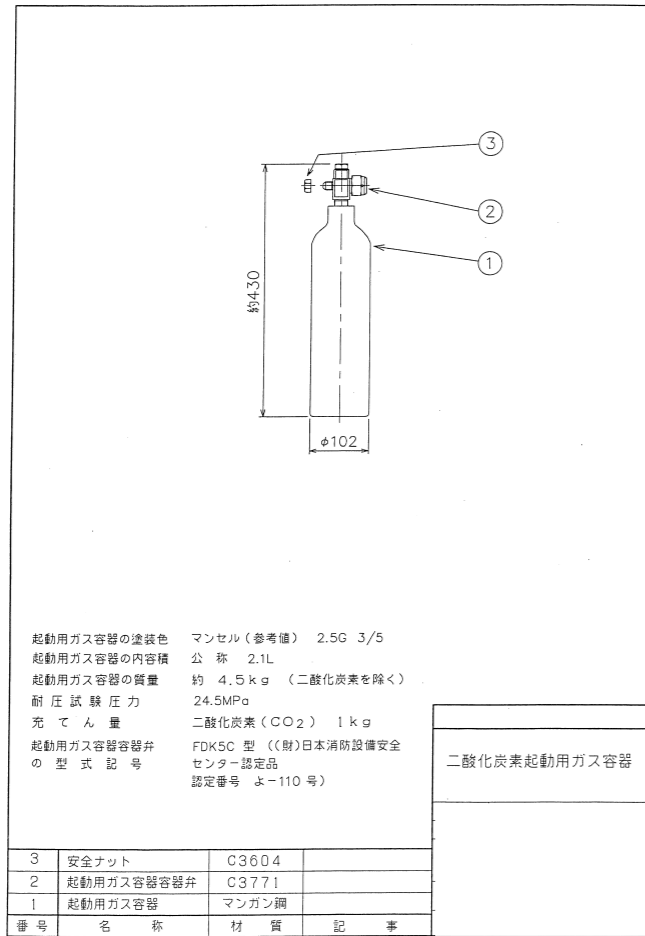
三国山起動容器姿図 S=1:N
