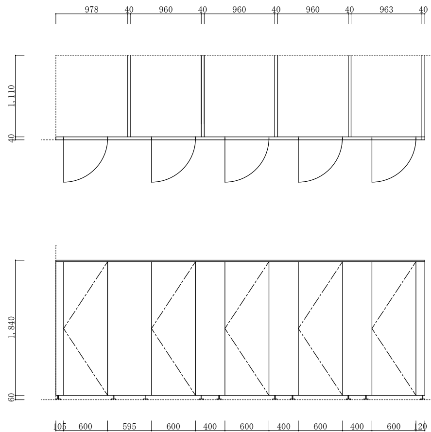
改修後トイレブース仕様
