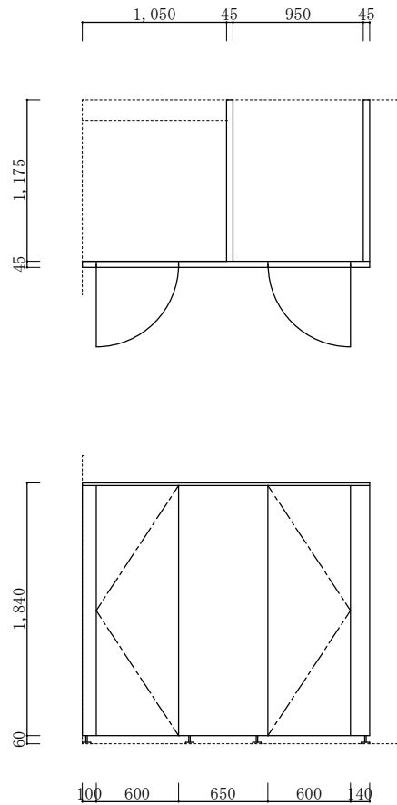
改修前トイレブース仕様
