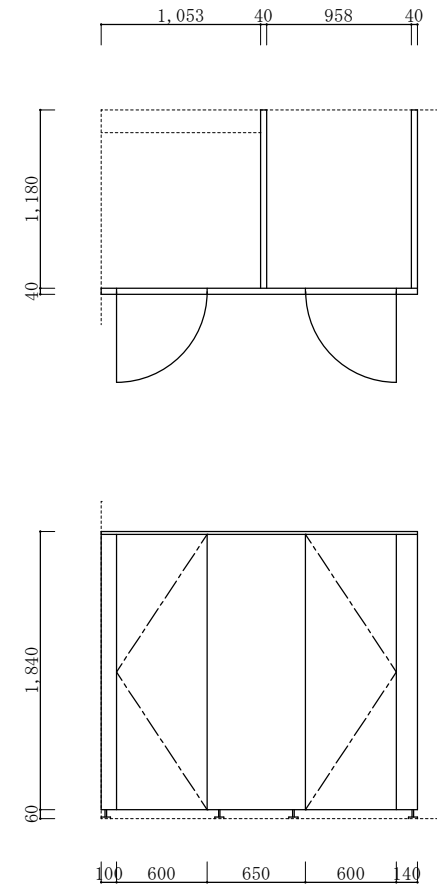
改修後トイレブース仕様
