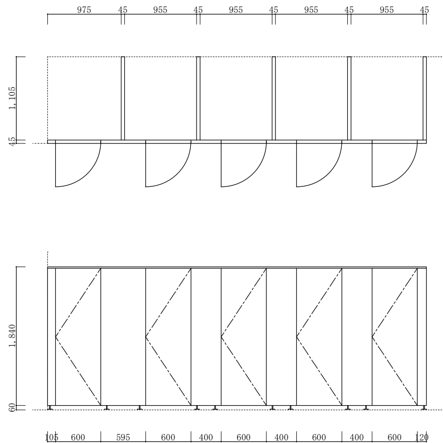
改修前トイレブース仕様
