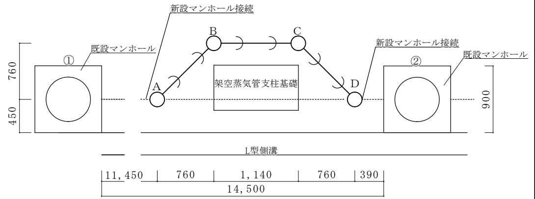
既設污水配管図 S = 1 / 5 0
