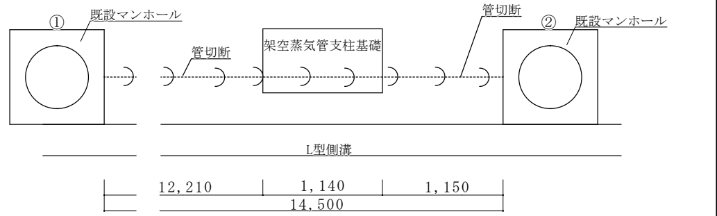
既設污水配管図 S = 1 / 5 0
