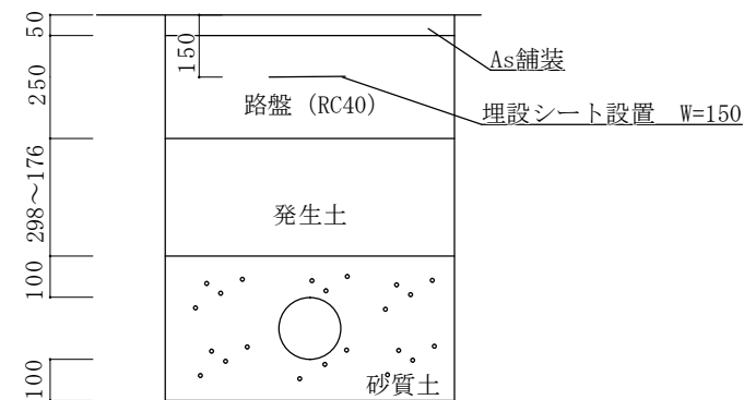
管路土工標準図 S=1/20
