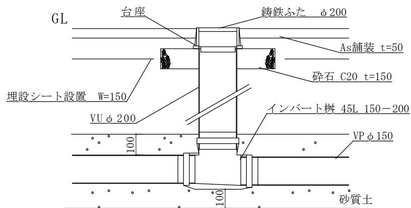
新設マンホール詳細標準図 S=1/20
