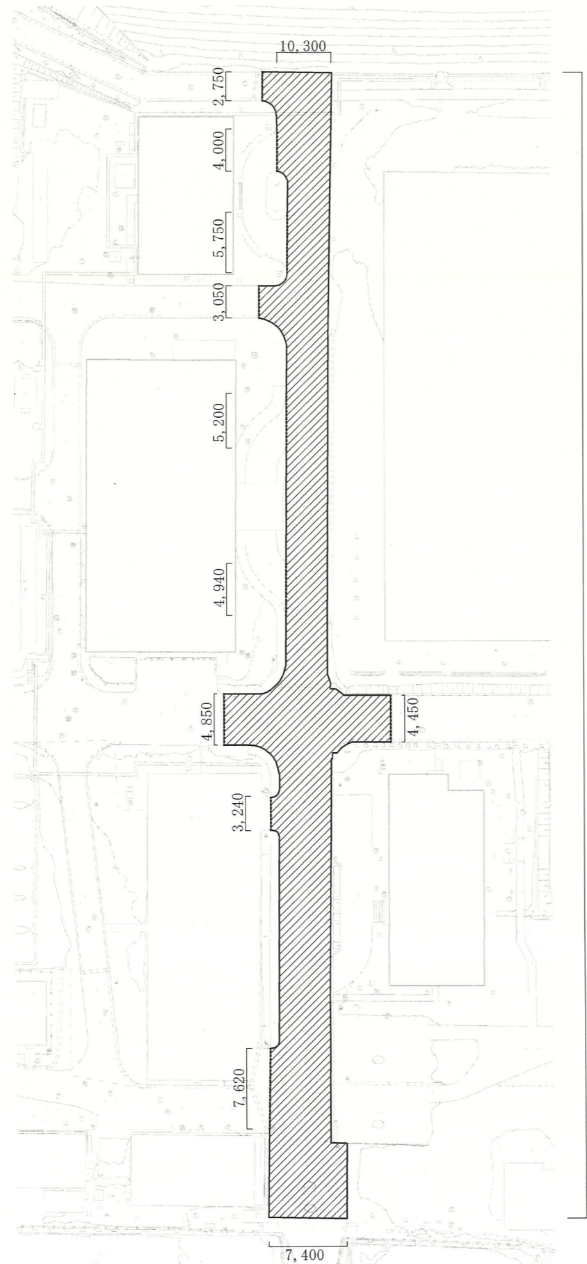
構内道路舗装施工箇所 S=1/1,000
