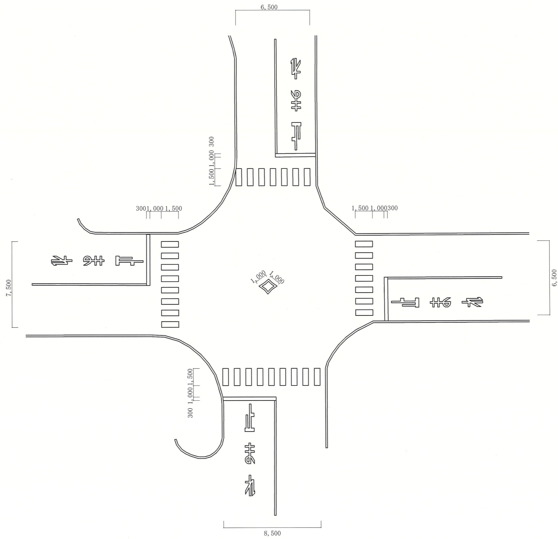
四又路施工箇所拡大図 S=1/200
