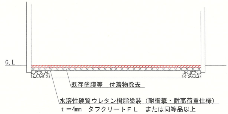
施工断面図 1/300
