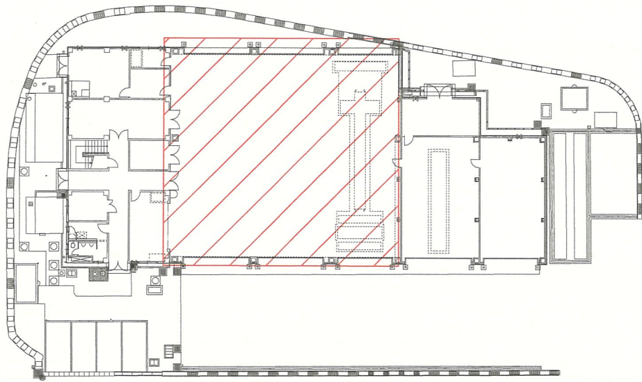
車両整備工場配置図 1/500
