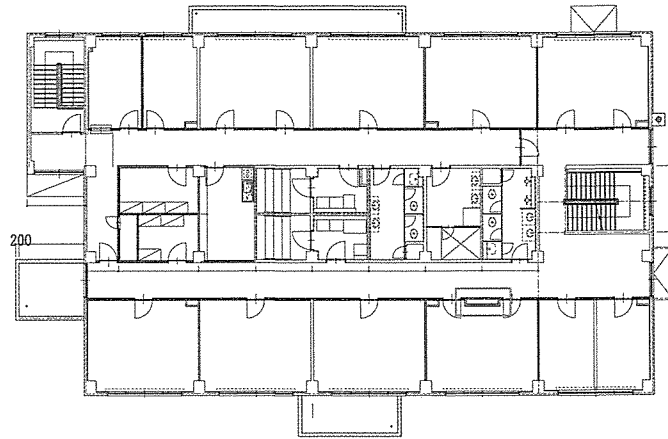
合棟隊舎 2階平面図 S = 1 : 500
