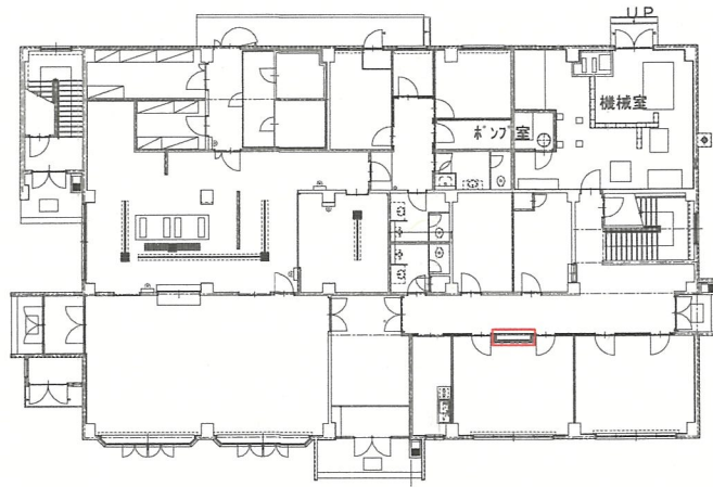
合棟隊舎1階平面図 S=1:500
