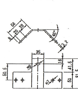
コーナープレート (隅柱部品)
