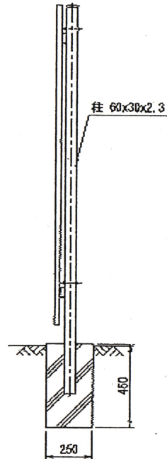
側面図 (S=1/20)
