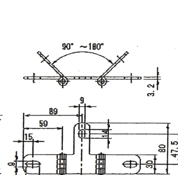
傾斜コーナー自在金具 (自在隅柱部品)
