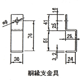
正面図 (S=1/20)
