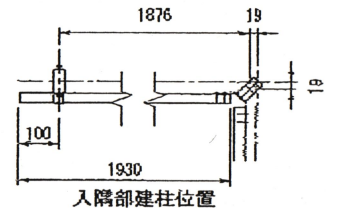
入隅部建柱位置
