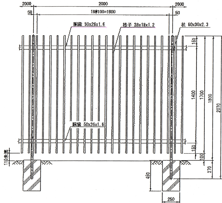
正面図 (S=1/20)
