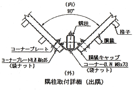
隅柱取付詳細 (入隅)
