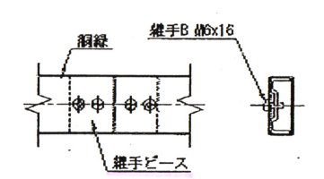
欄縁・継手取付詳細
