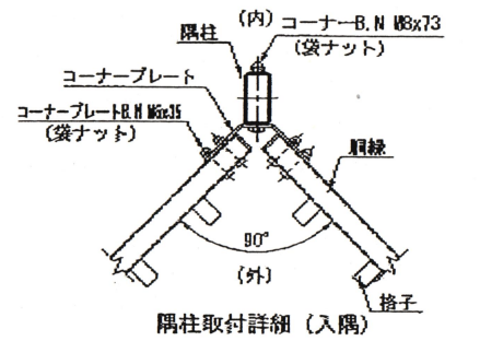
柱・欄縁取付詳細
