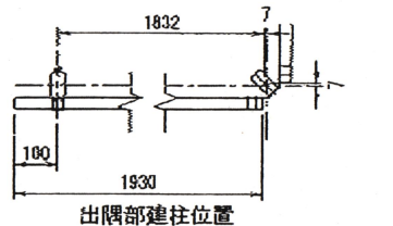
出隅部建柱位置
