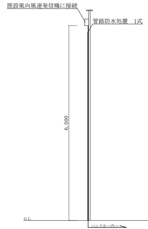
風向風速発信器支柱 S=1/60
