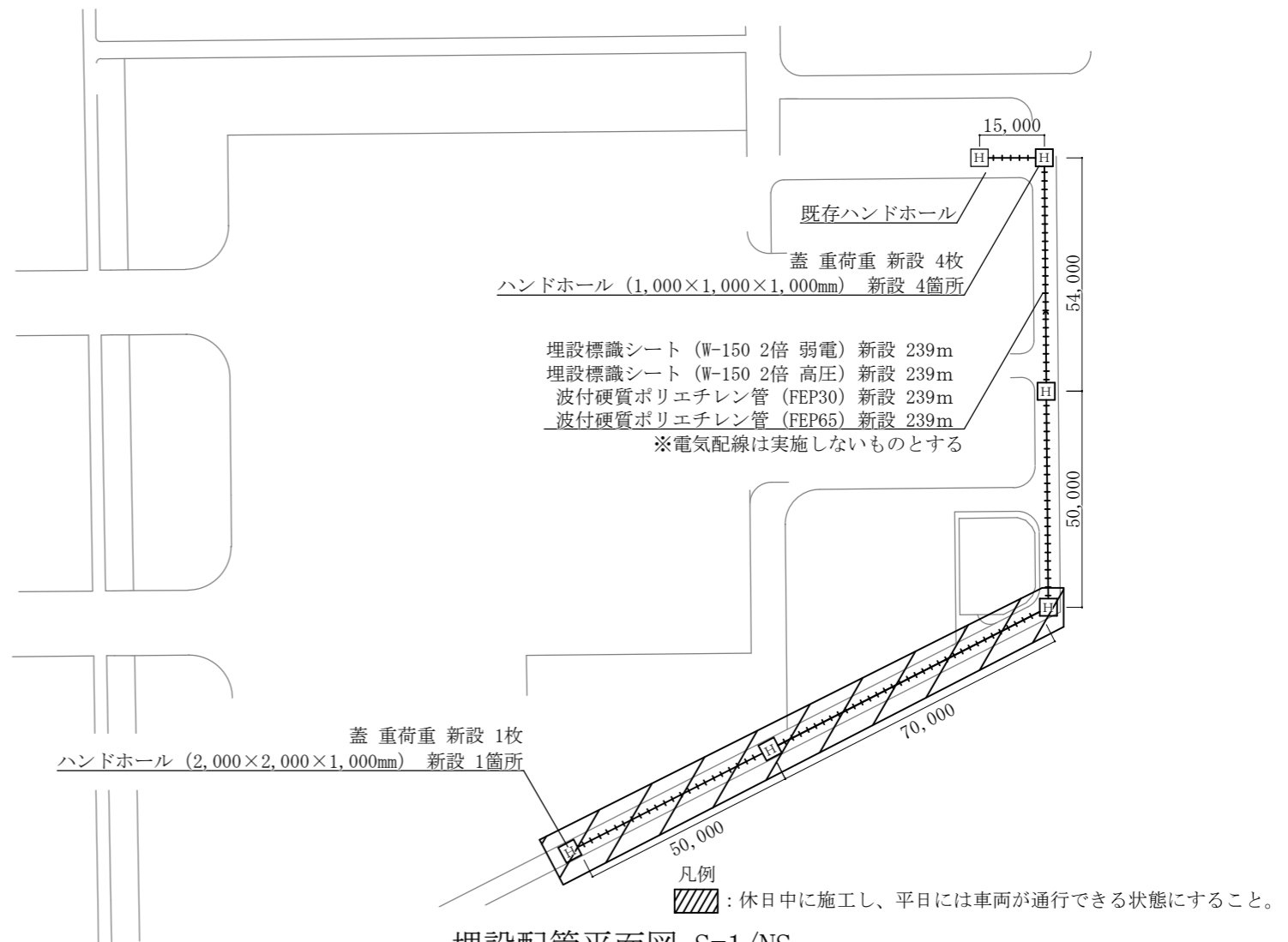
埋設配管平面図 S=1/NS
