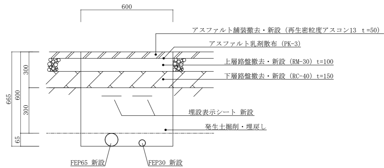
埋設配管掘削詳細図 1/NS
