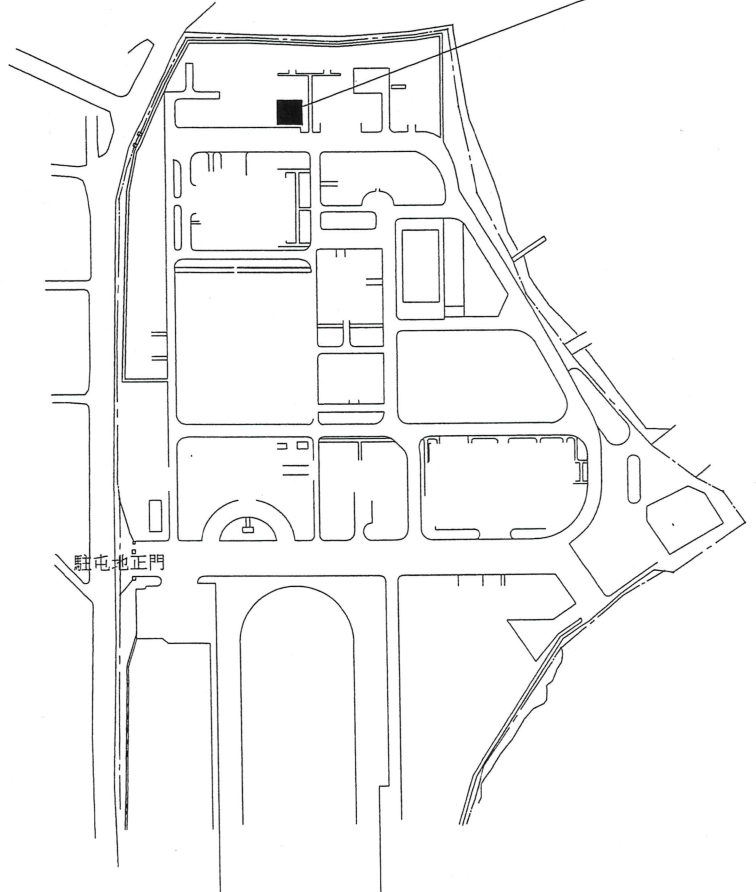
配置図 S=1/3,000
