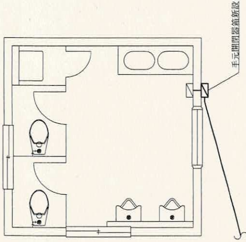
1 2 3号建物平面図 S=1:50
