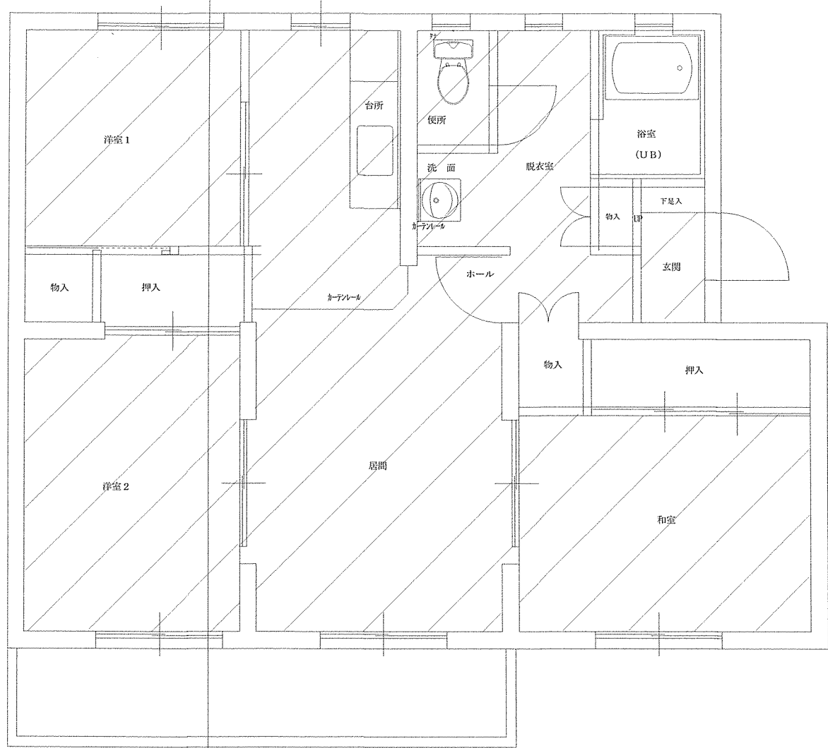
白国宿舎平面図 1:50
