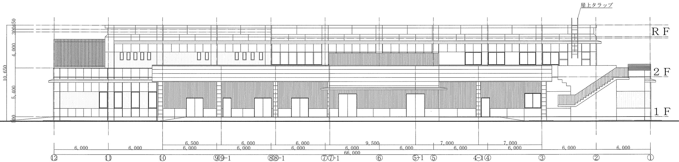
北側立面図 S=1/400
