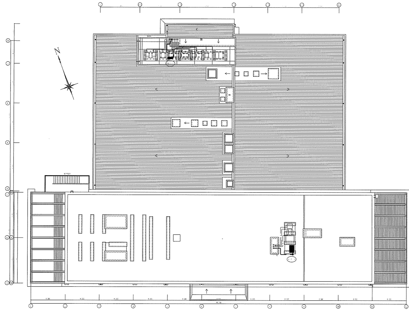
屋上空調設備配置図 S=1/400
