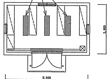
260号建物平面図 (S=1:100)
