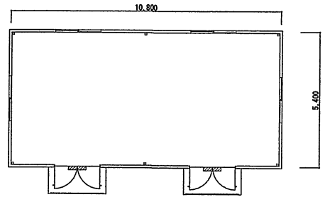
258号建物平面図 (S=1:150)
