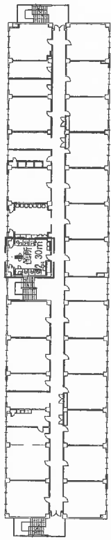
4階平面図 S=600
