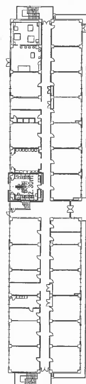
1階平面図 S=600
