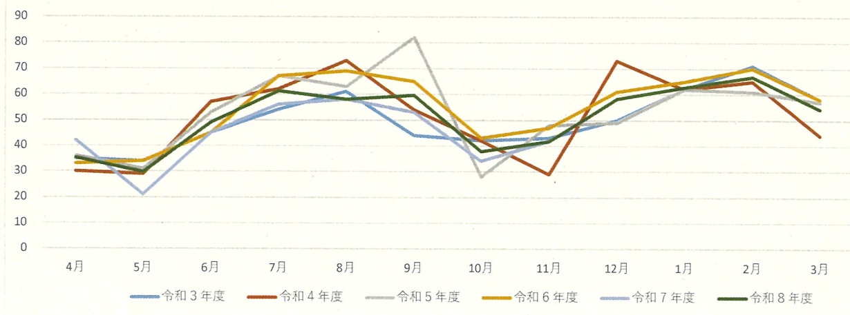
最大需要電力量比較グラフ
