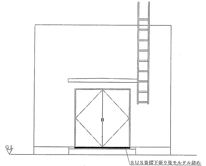
鋼製扉設置状況 S=1/60
