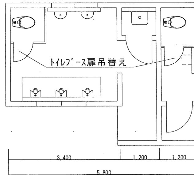
154号便所改修後平面図
