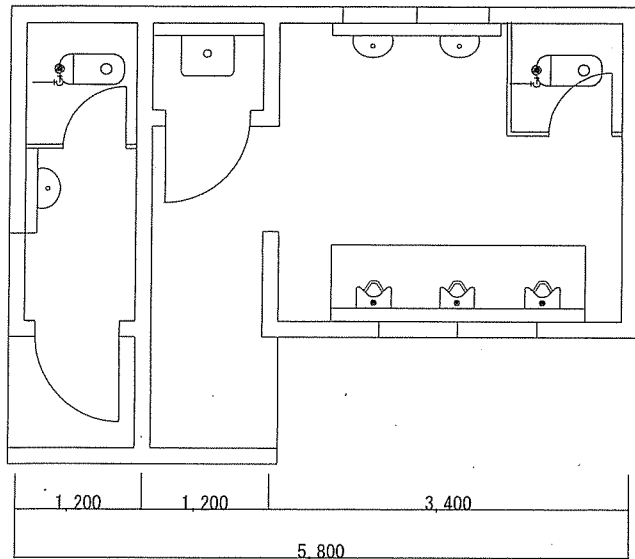
153号便所改修前平面図
