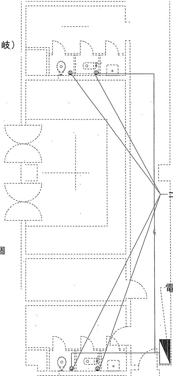
5号2階 電気改修平面図
