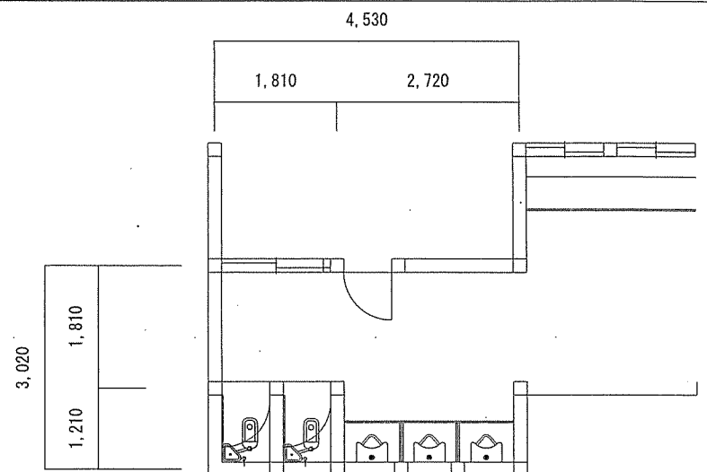
88号便所改修前平面図
