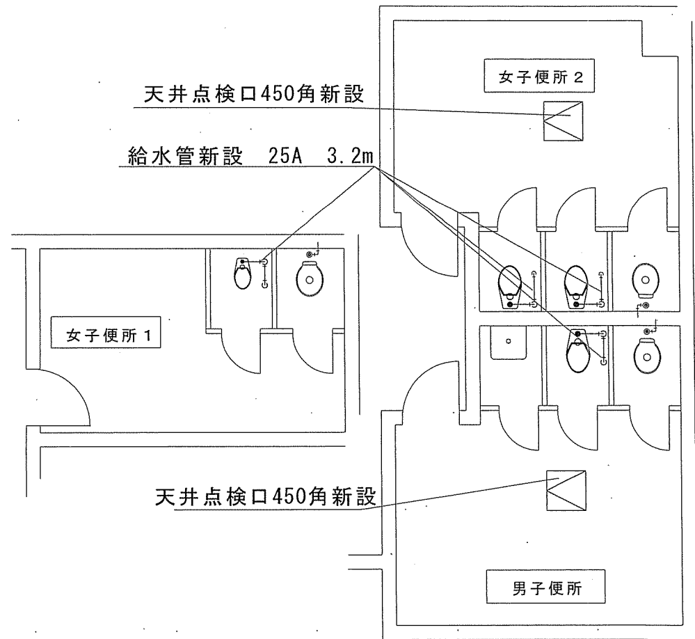
5号1階便所改修後平面図
