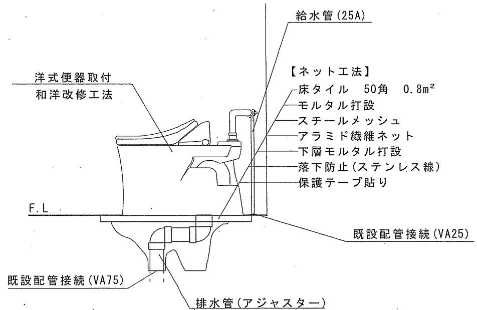
改修標準図 S=1/20
