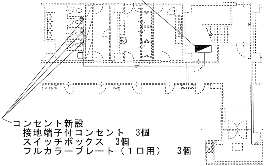
10号1階 電気改修平面図
