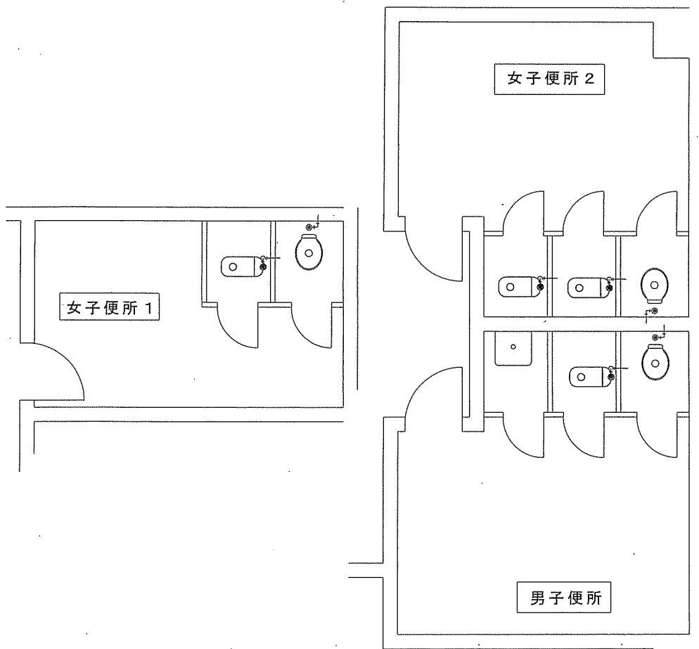
5号1階便所改修前平面図
