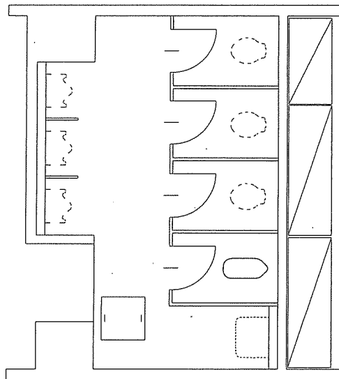
10号1階便所改修前平面図
