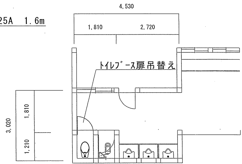
88号便所改修後平面図
