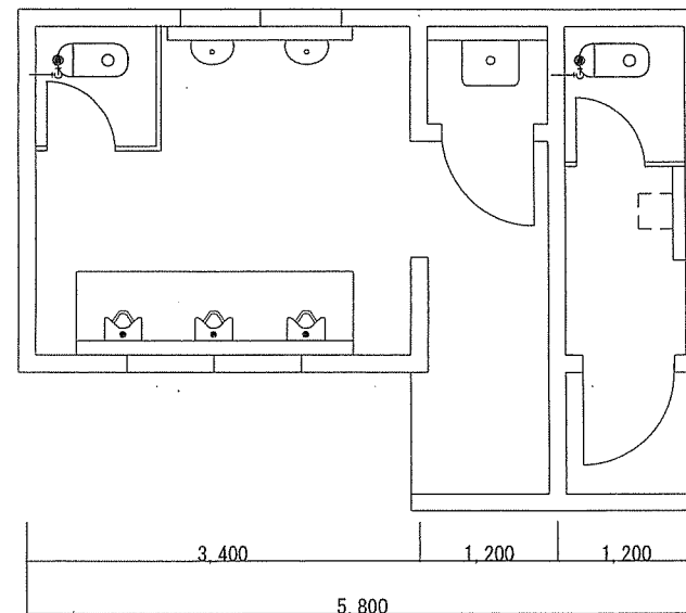
154号便所改修前平面図
