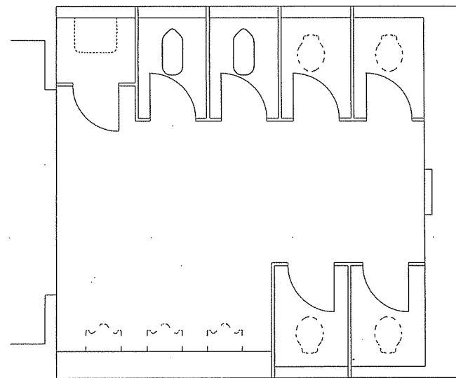
10号3～5階便所改修前平面図
