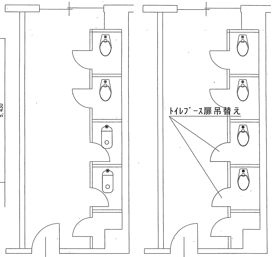
8号1~4階便所改修前平面図
