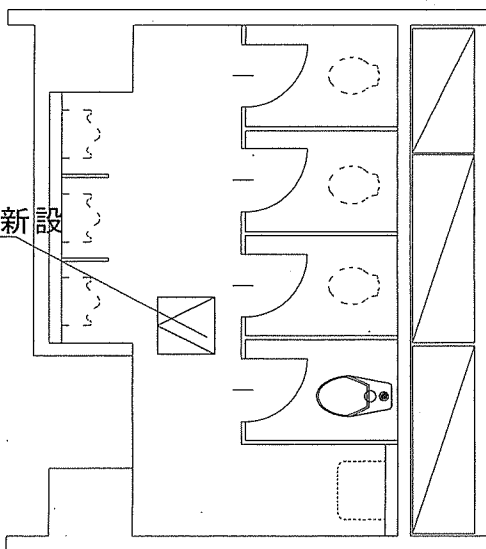
10号1階便所改修後平面図
