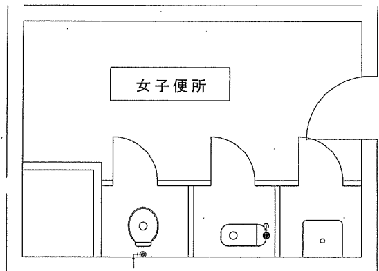
5号2階便所改修前平面図
