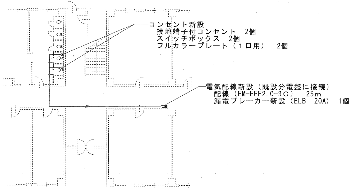
8号1~3階 電気改修平面図
