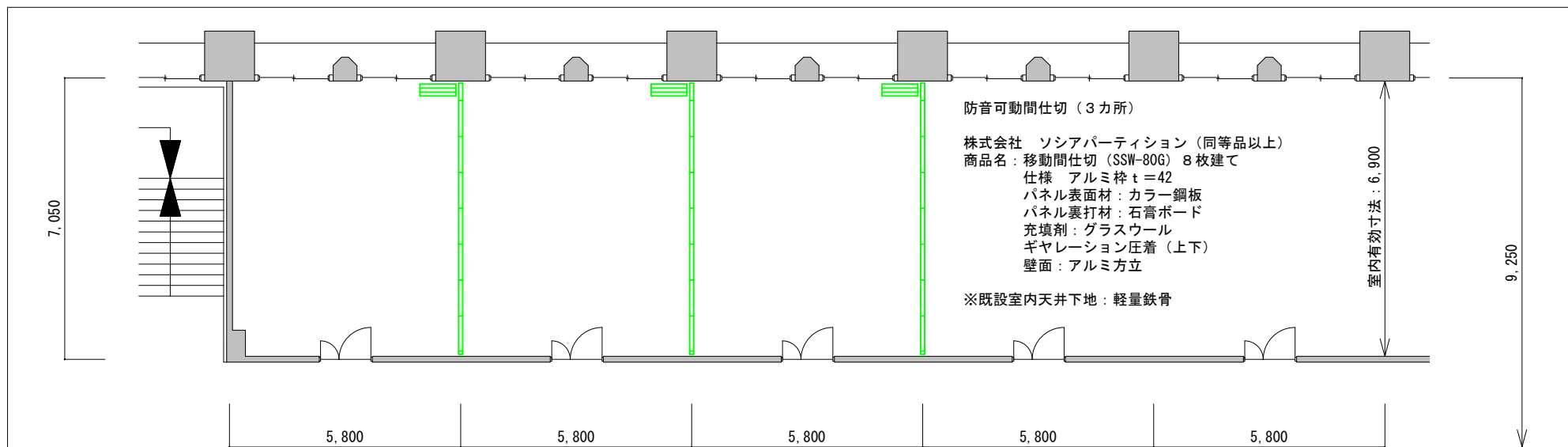
間仕切壁取付位置 S=1/150
