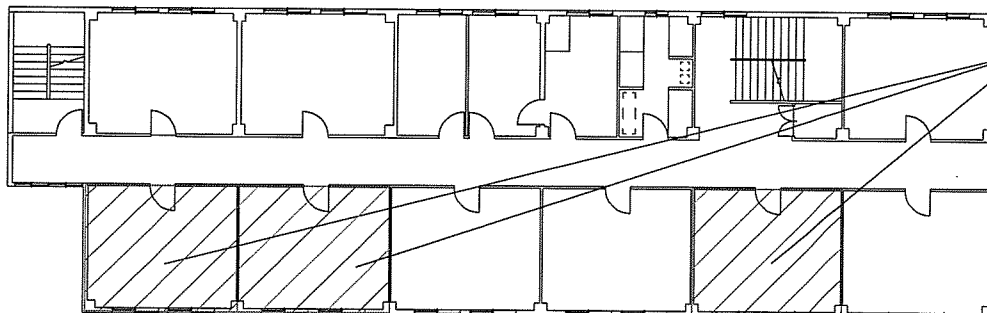
23号生活隊舎2階平面図
