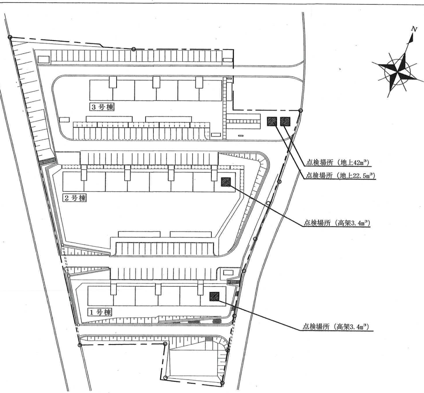
滝本宿舎配置図 S=N/1000
